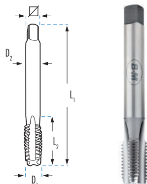
FILETTATURA CONICA AMERICANA PER TUBI
