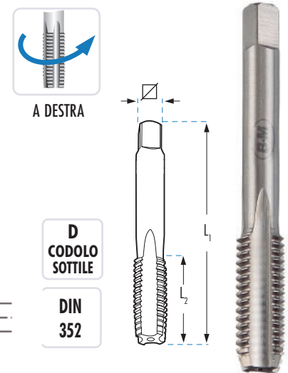
Ref. M03: Cono di entrata 2-3 filetti
