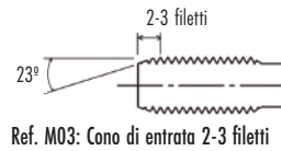
Ref. M03: Cono di entrata 2-3 filetti
