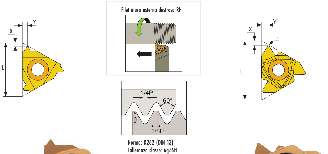
Profilo parziale
